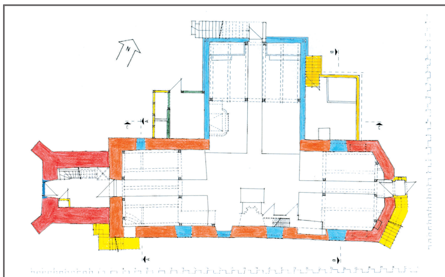
3 Warmsen, Ldkr. Nienburg, St. Georgskirche, Baualtersplan (vorläufig).
