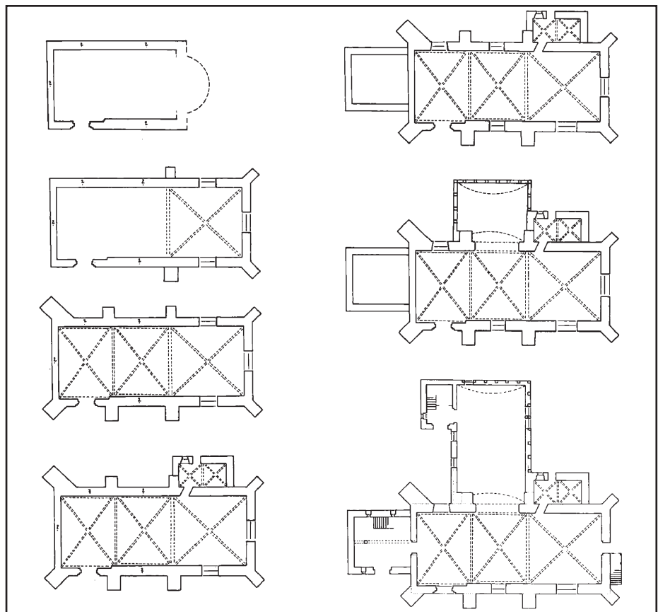
2 Steyerberg-Rießen, Ldkr. Nienburg, St. Katharinen-Kirche, Bauphasenplan, links von oben nach unten: mittelalterliche Bauentwicklung, rechts: oben 1507, Mitte 1737, unten 1908.
